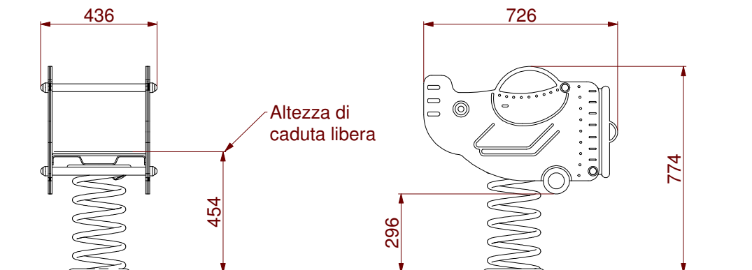
FRONTE
